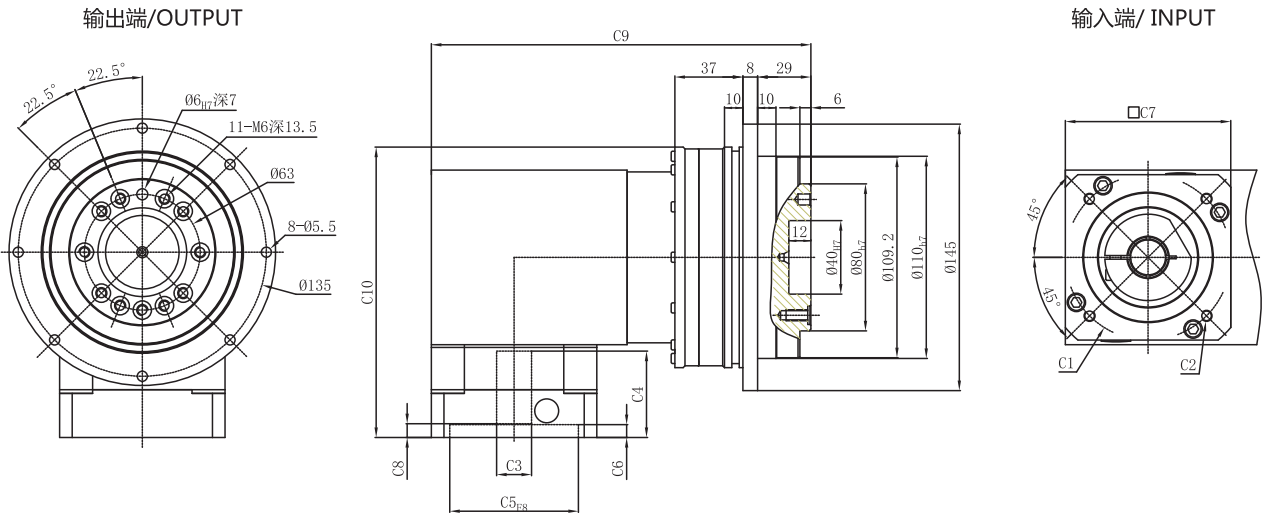
PGFR 110-L2
