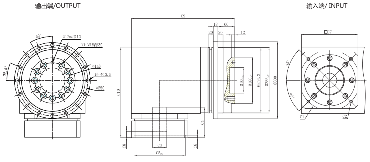
PGFR 255-L1
