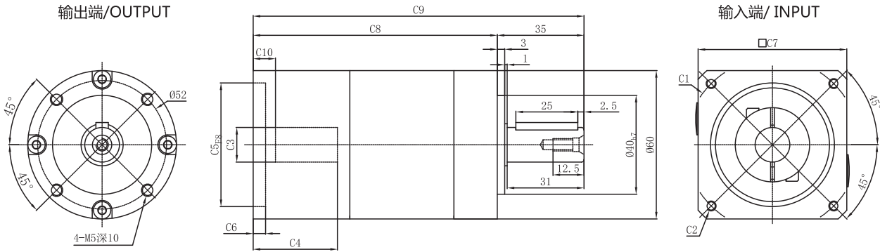
PGC060-L2
