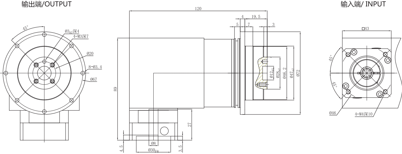
PGFR 047-L2
