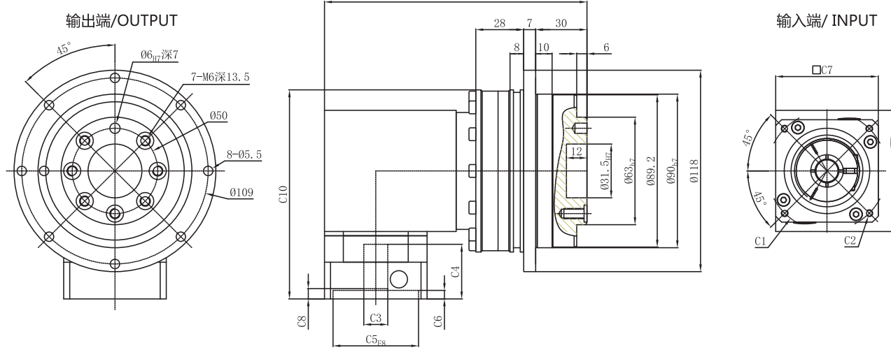
PGFR 090-L2
