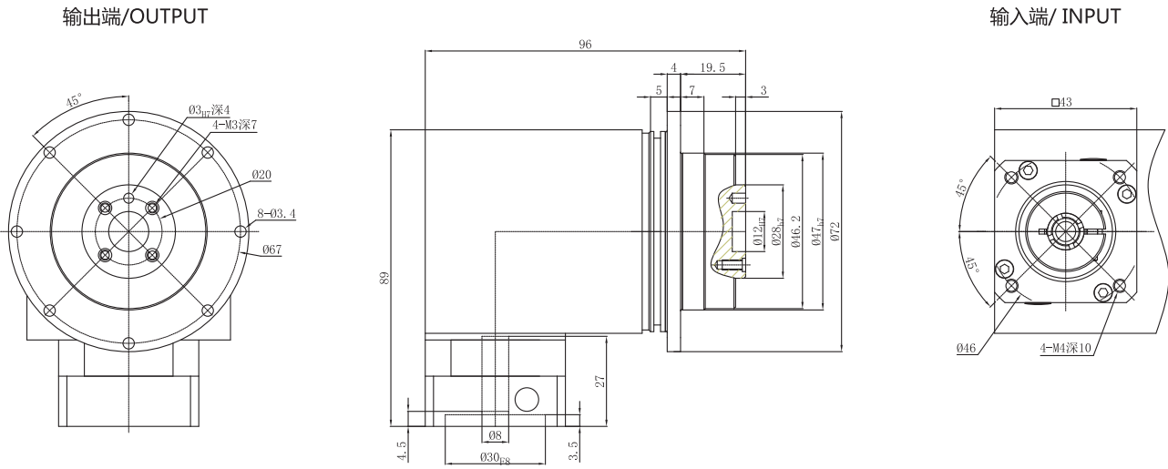
PGFR 047-L2
