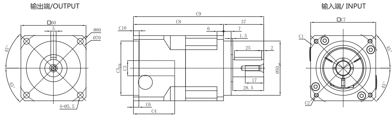
PGL060-L1
