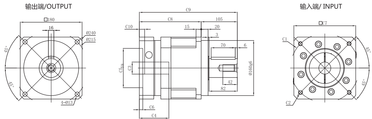
PGH180-L2
