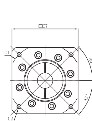
输入端/INPUT
