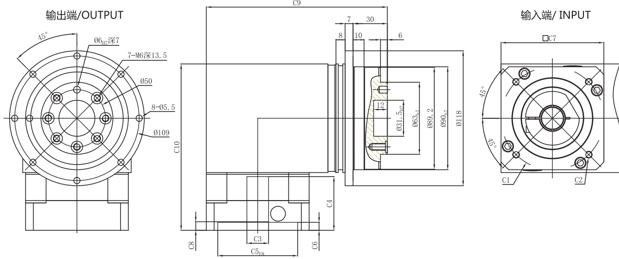
PGFR 090-L2
