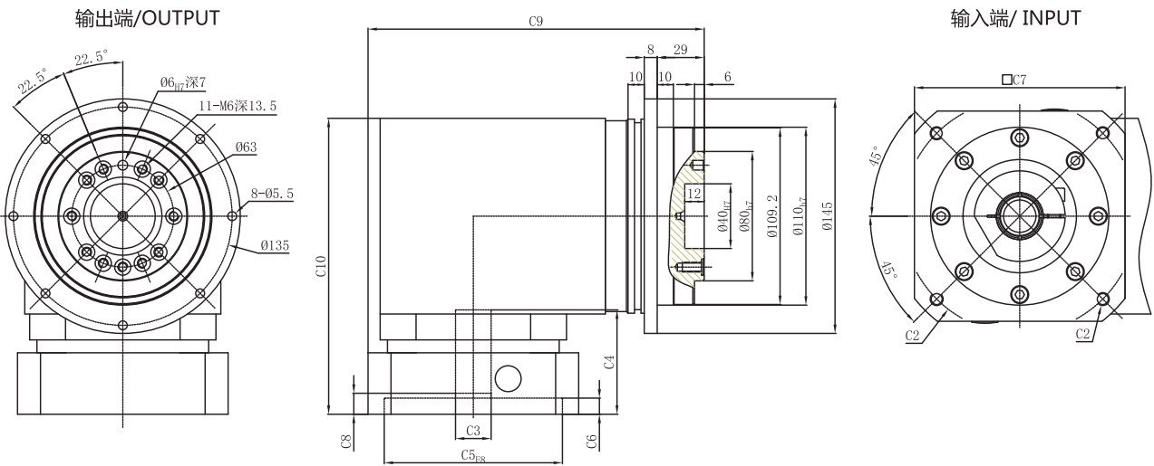
PGFR 110-L1
