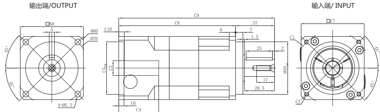
PGL060-L2
