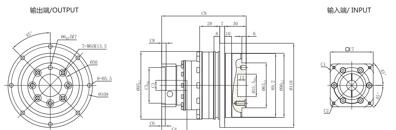
PGF090-L2
