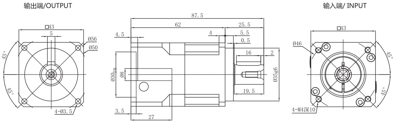
PGH042-L2
