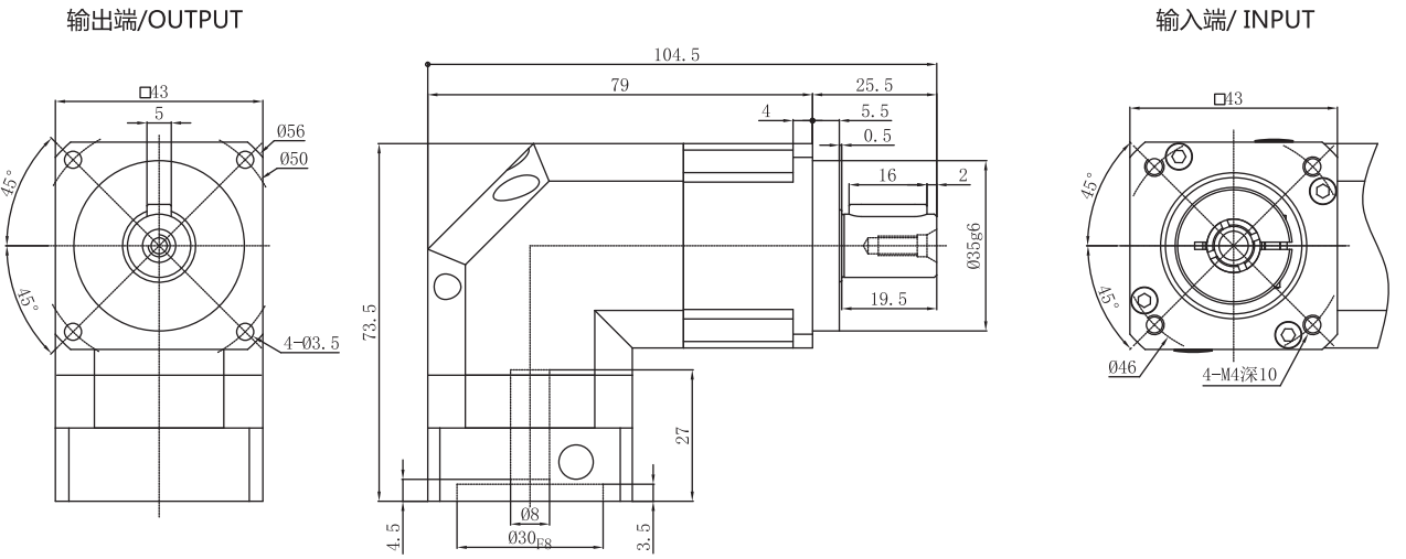
PGHR042-L2
