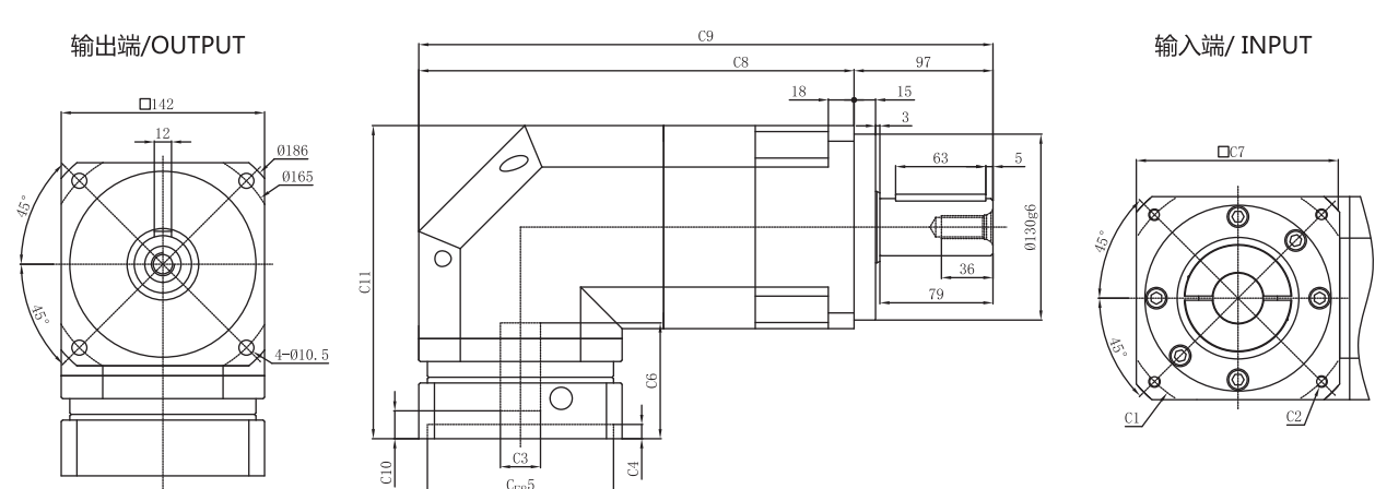
PGHR142-L2
