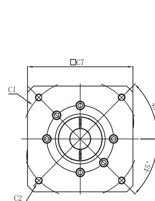
输入端/INPUT
